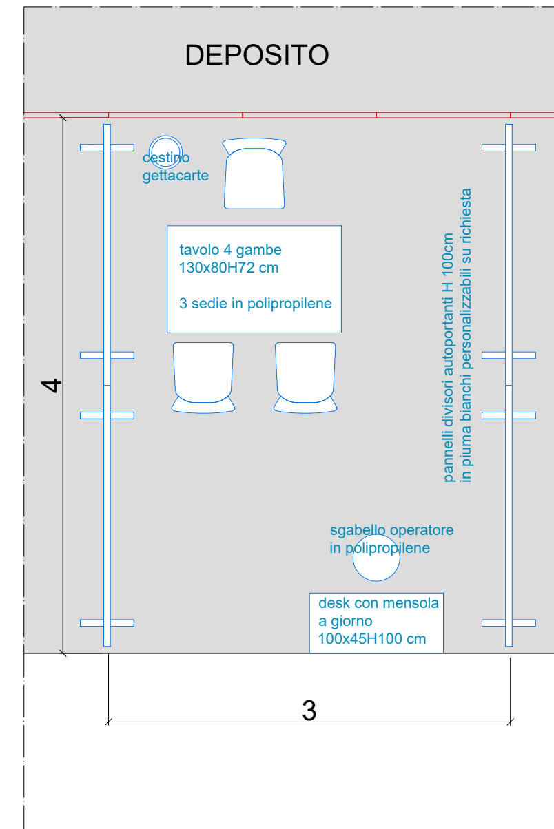
planimetria stand - tipo di 3x4m
